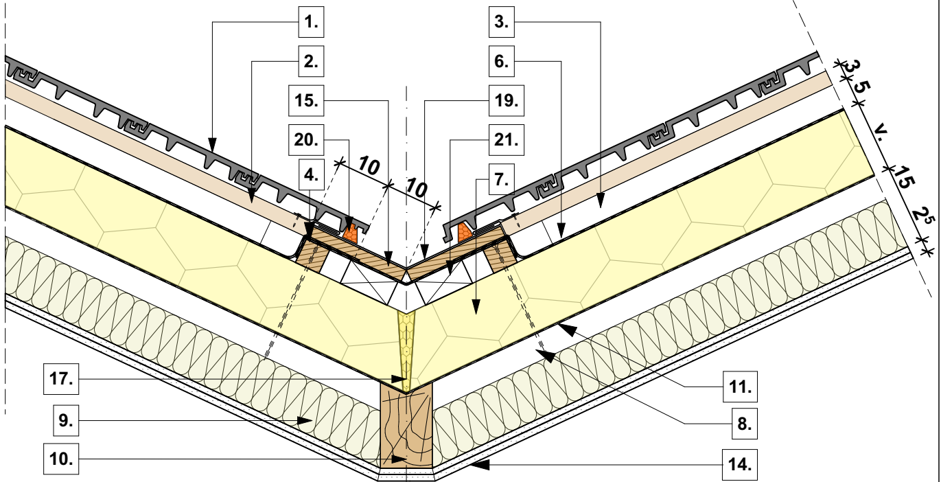
Orom részletrajz
