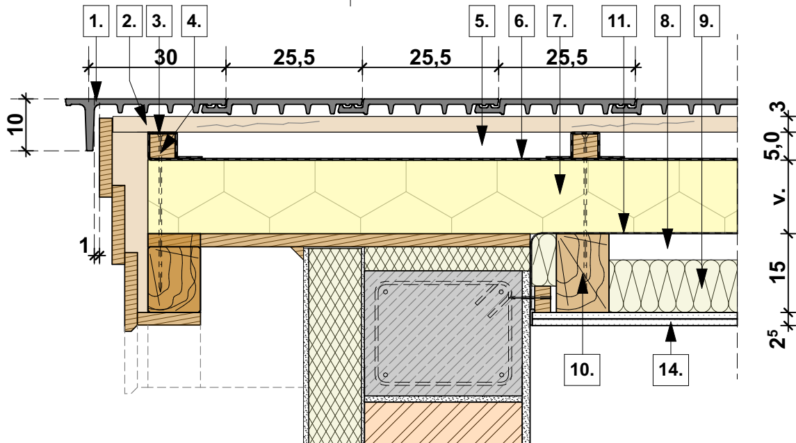
Orom részletrajz
