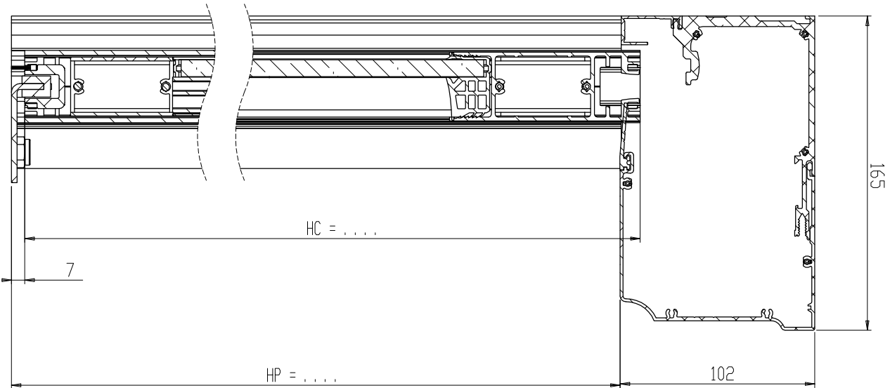
COUPE B-B ECHELLE 1 : 2
