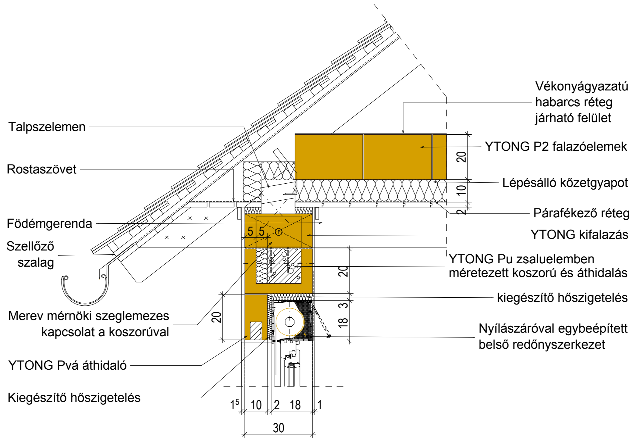
Belső redőnyszerkezt beépítési példa 30 cm-es falba, tárcsamerev pór-fafödémme
