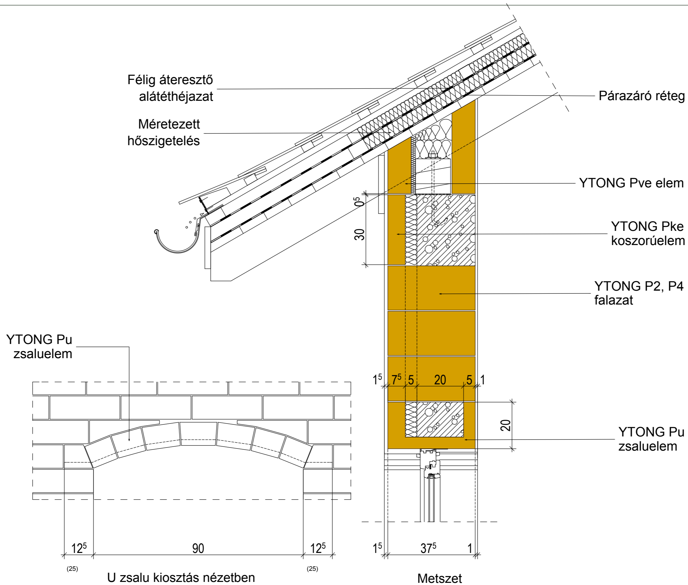
12. Ereszcsomópont vb. vázas közösségi funkciós térnél Íves "U" zsalus áthidalással
