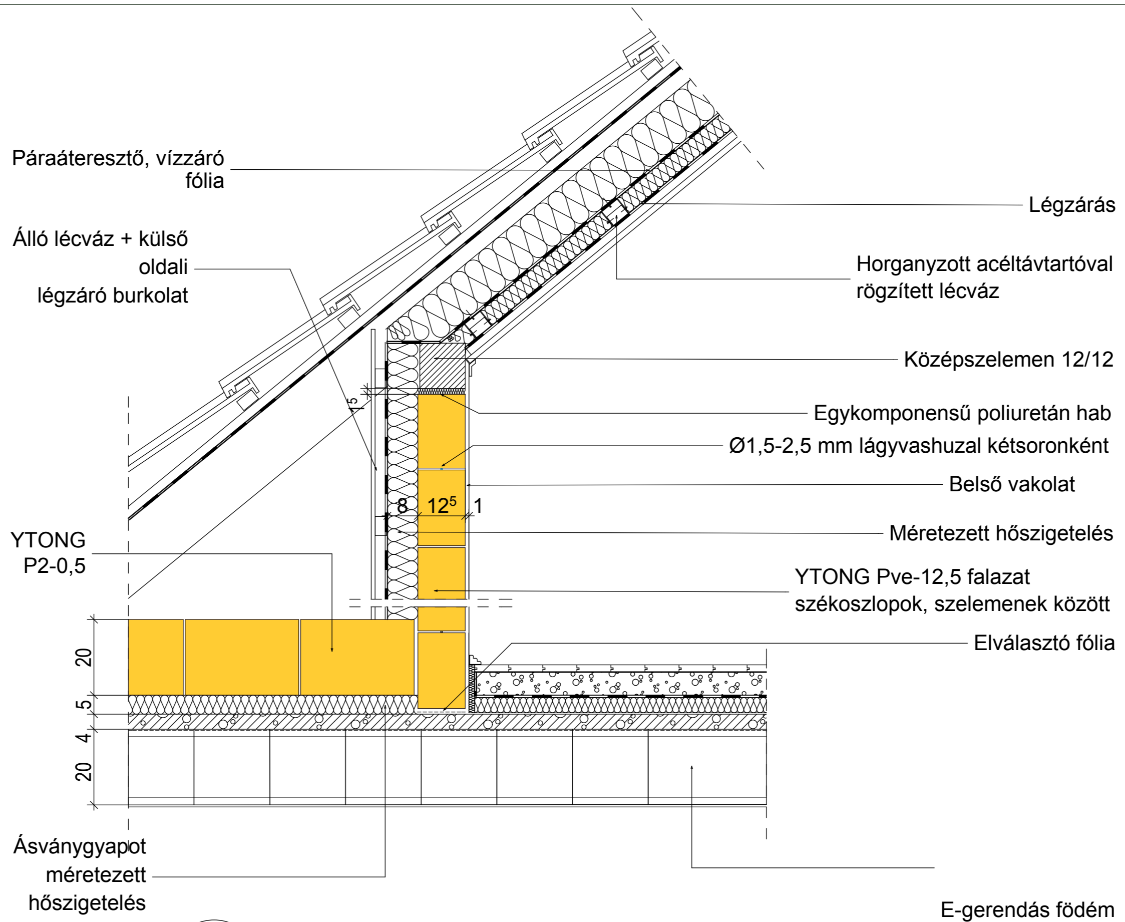
Példa tetőtéri térdfal beépítésére függőleges metszet
