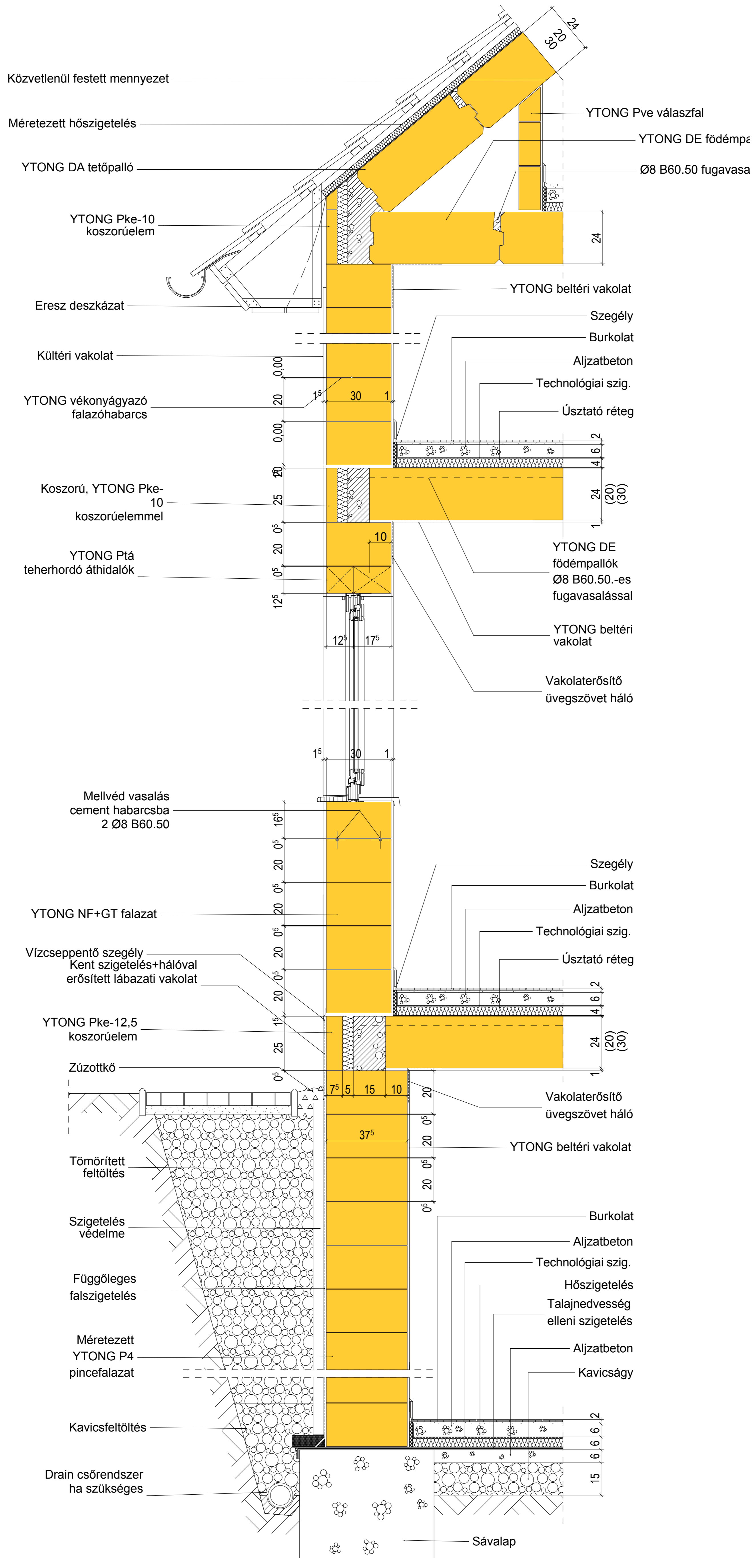
19. Függőleges falmetszet
