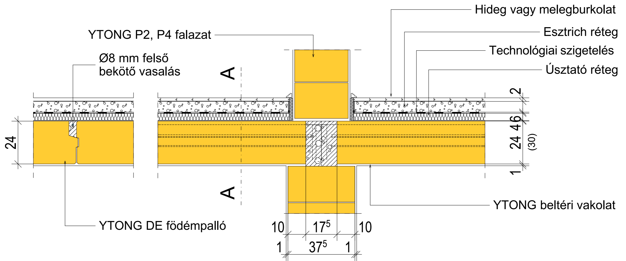
A - A metszet
