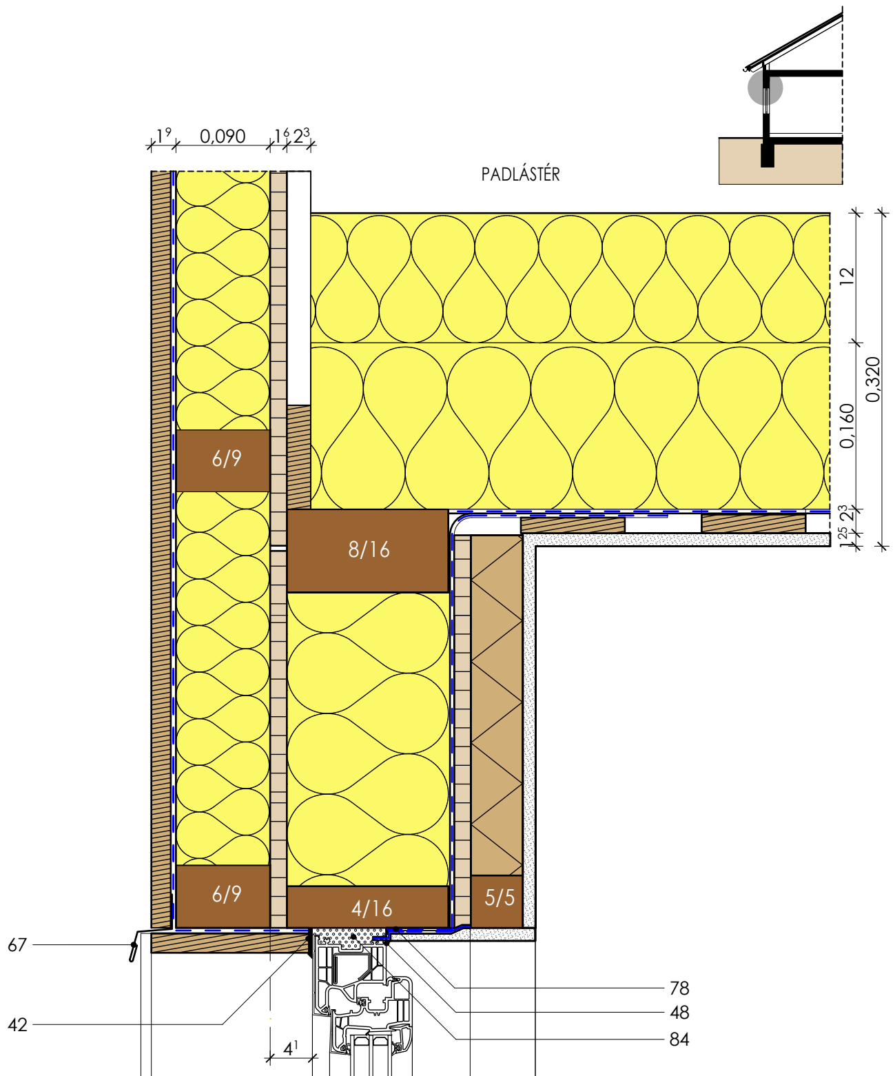
ABLAK SZEMÖLDÖK CSOMÓPONT homlokzati faburkolatnál, redőny nélkül M= 1:5
