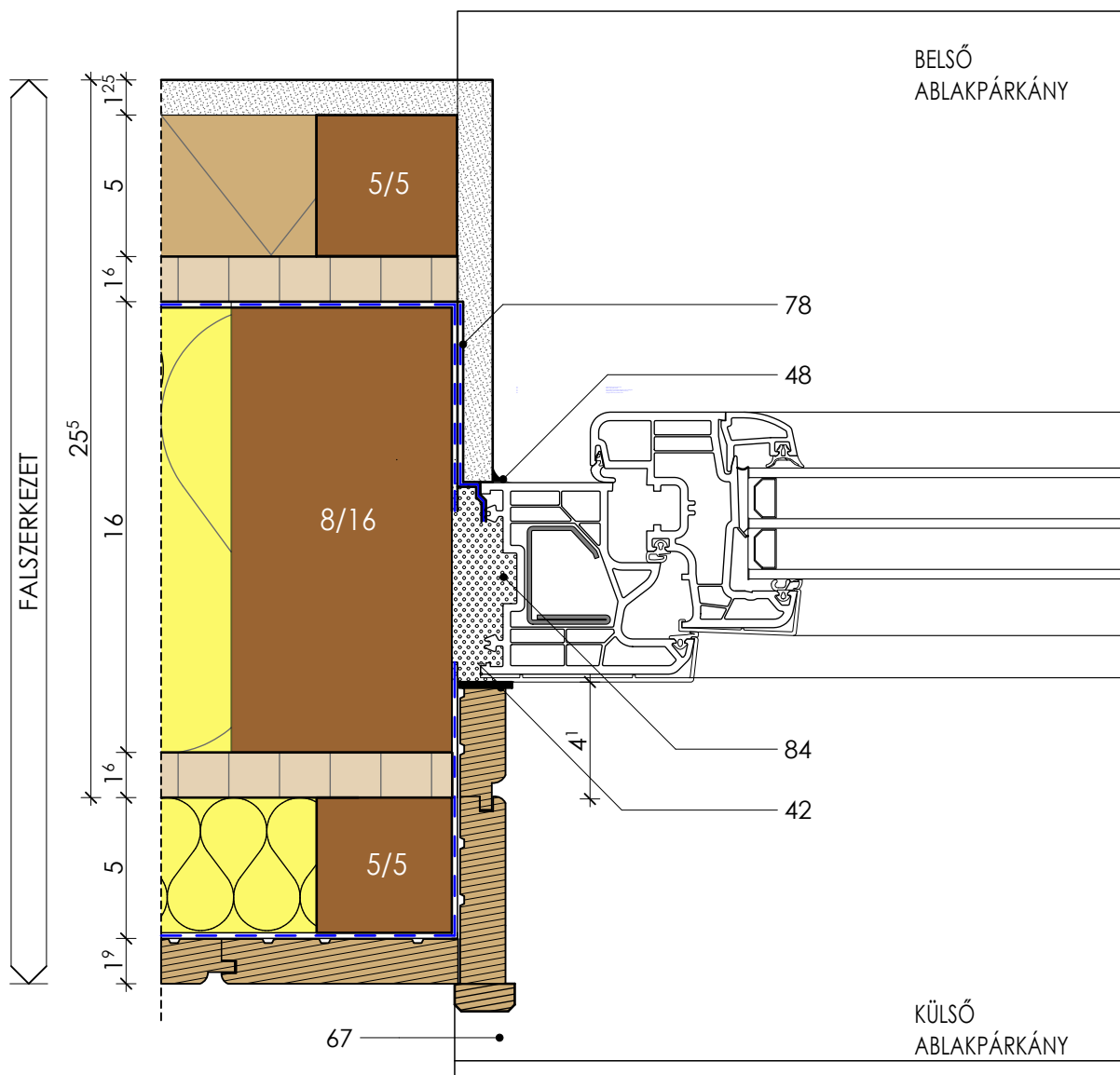
ABLAK VÍZSZINTES METSZET redőny nélkül M= 1:2,5
